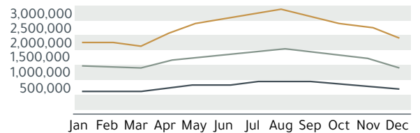
استهلاك الطاقة شهرياً (كيلوواط/ساعة) لمبنى بورصة الكويت
